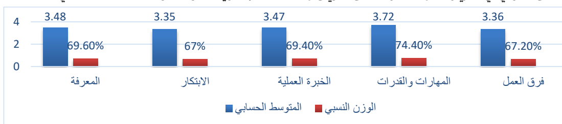
الشكل رقم (2). المتوسط الحسابي والوزن النسبي لمحاور متغير (رأس المال الفكري) X1
