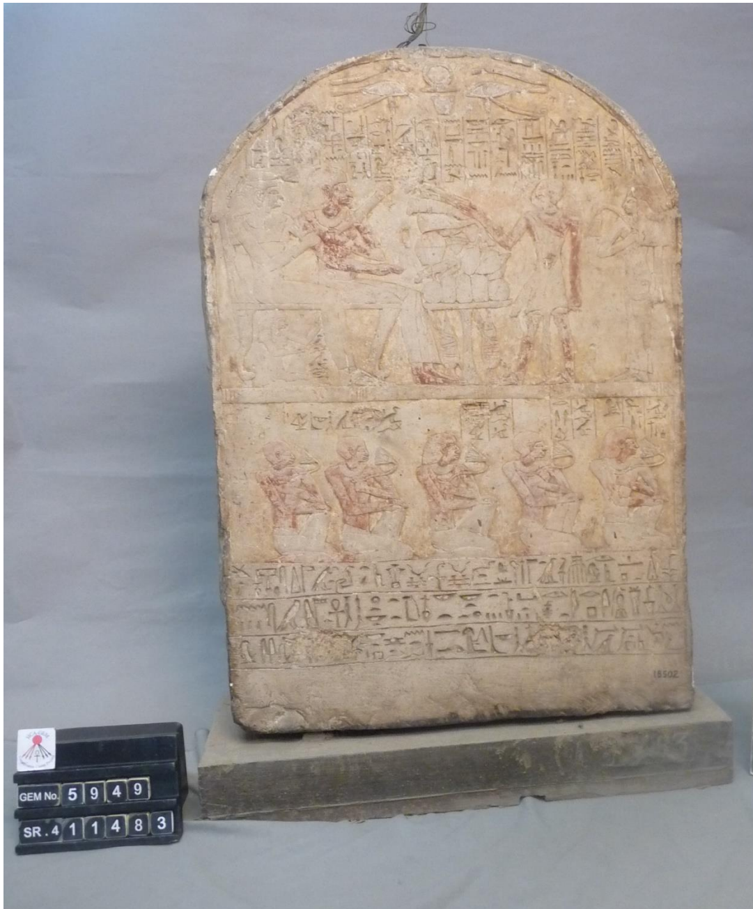
Pl. 2 stèle CG 34.101
