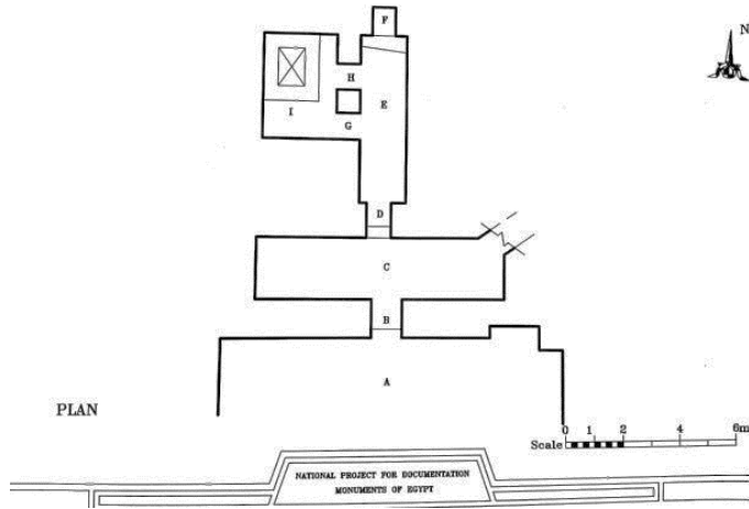
شكل رقم 3: تخطيط المقبرة
