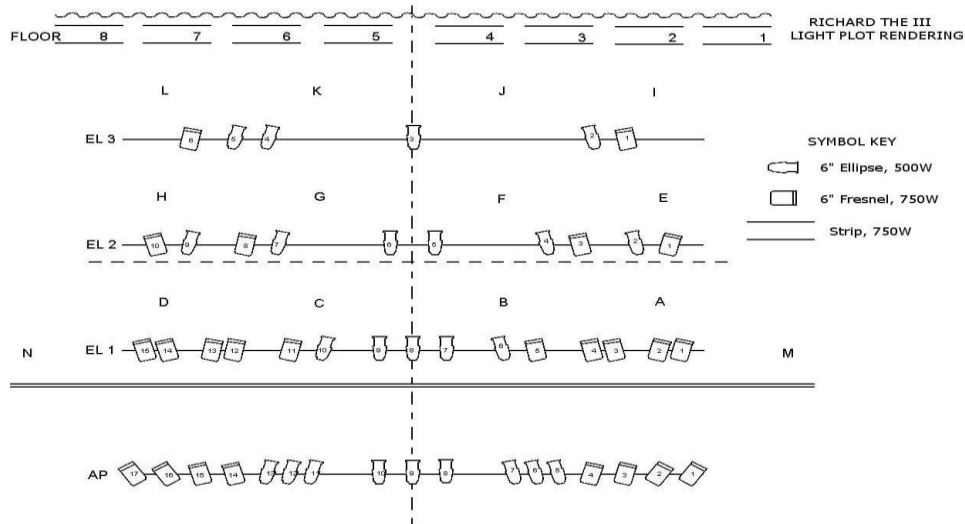
شكل (١) نموذج لمسقط أفقي يوضح أماكن الهريس و مثبت عليها أجهزة الإضاءة المسرحية
