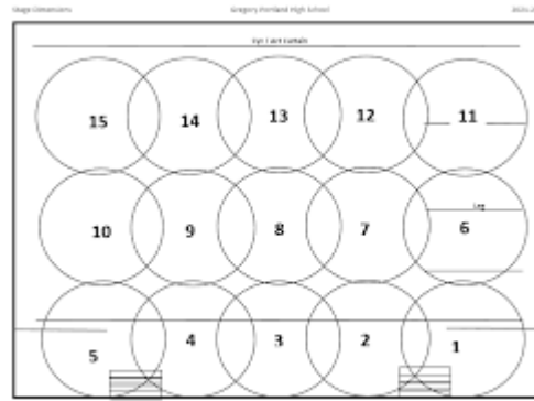
شكل (٢) نموذج لمسقط أفقي يوضح مواقع الإضاءة على خشبة المسرح
