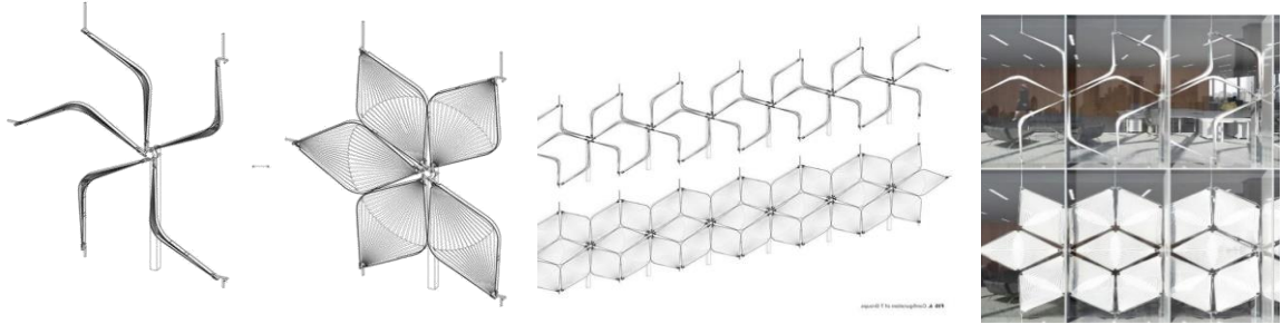
شكل (١٢) الفواصل الزجاجية معيارية وطرق تركيبها
