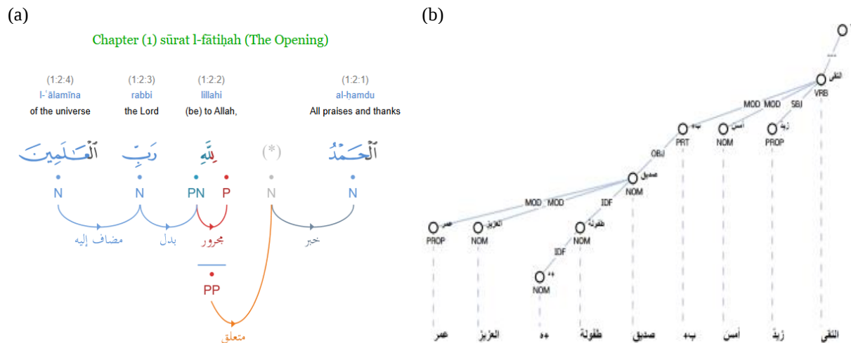
Figure 9 : un exemple de graphe de dépendance issue de Quranic Arabic Corpus et arbre de CamelTB
