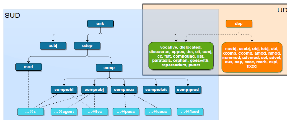
Figure 2 : le schéma des relations syntaxiques employées dans SUD issu de Gerdes et al. (2019a)
