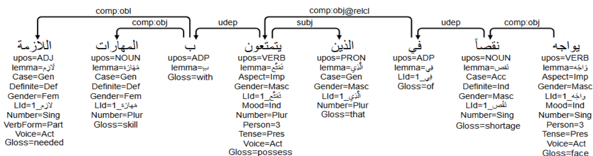
Figure 21 : l'analyse proposée dans SUD
