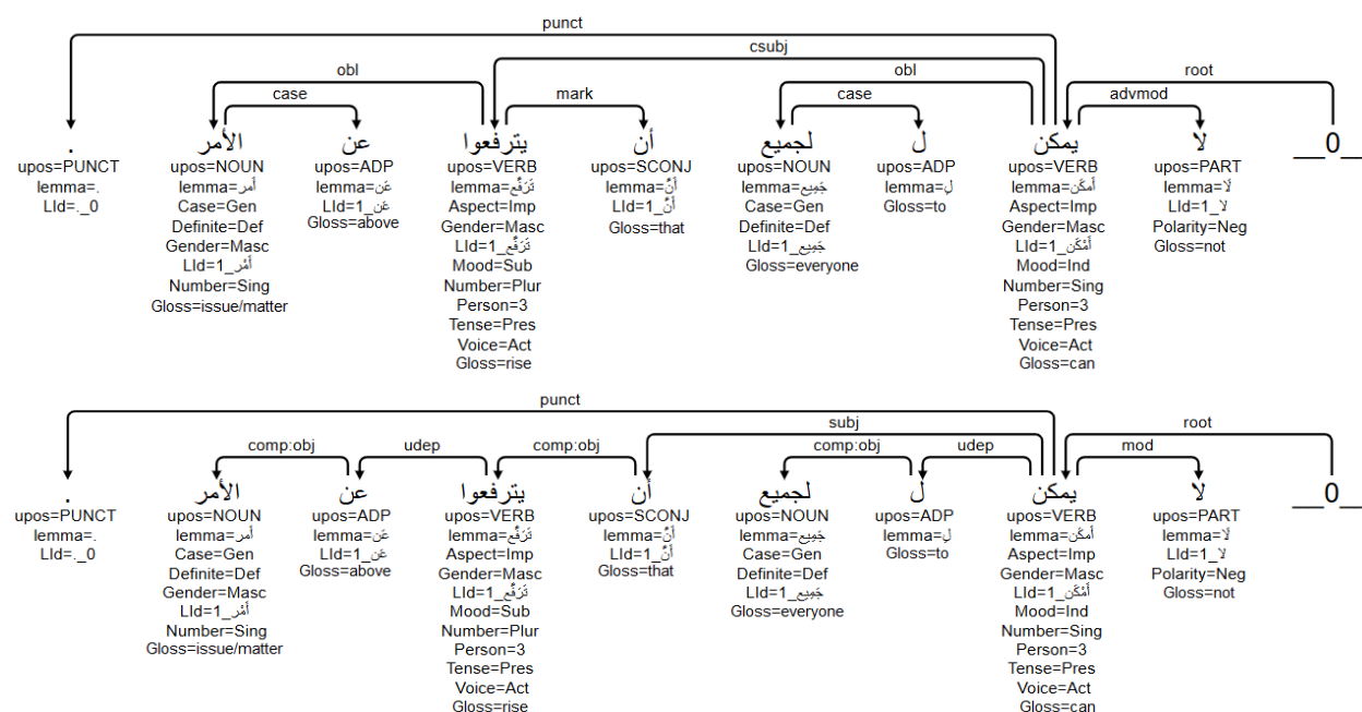
Figure 1 : l'annotation morphosyntaxique UD (en haut) et SUD (en bas) pour la même phrase de l'arabe (' Tout le monde ne peut pas s'élever au-dessus de ça '), tiré du treebank Arabic-PUD@2.15 4
