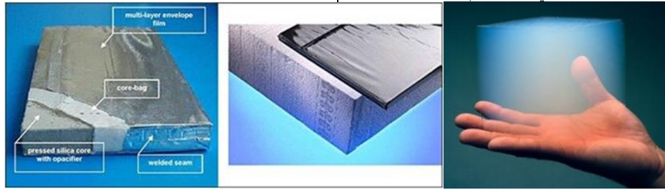
صورة توضح على اليمين مادة الايروجيل وعلي اليسار الألواح العزل المفرغة VIPS
