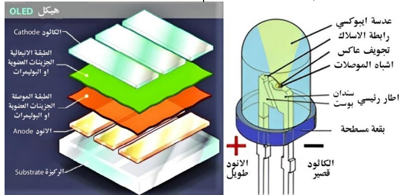
صورة ٣ توضح مكونات LED & OLED
