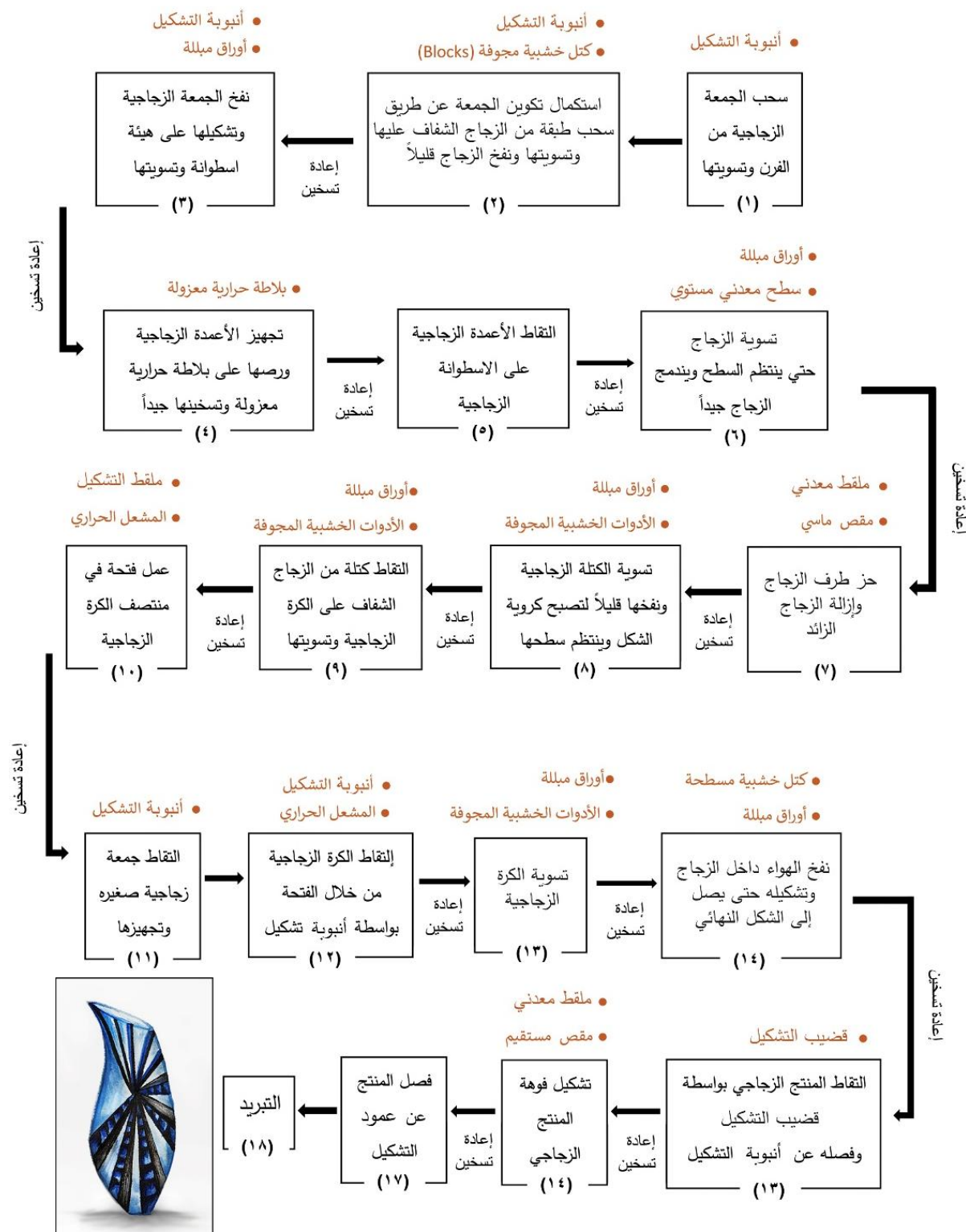
شكل (20) تخطيط العملية الإنتاجية لفازة زجاجية ذات مظهر لوني مستنبت من ريش طائر القيق الأزرق تُنفذ بتقنية التشكيل الحر
