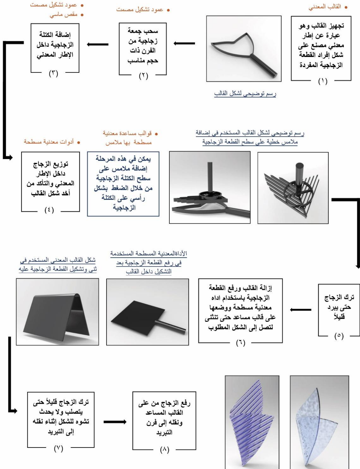
شكل (26) تخطيط العملية الإنتاجية لتنفيذ القطعة الزجاجية المفردة المستنبطة من طائر القيق الأزرق، مع تصميم القوالب المساعدة المستخدمة في التشكيل
