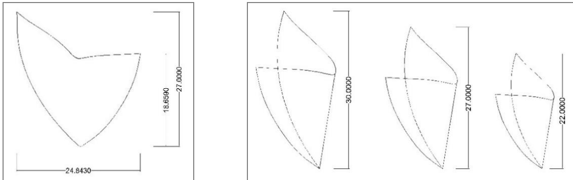
شكل (22) مساقط القطع الزجاجية المفردة وأبعادها
