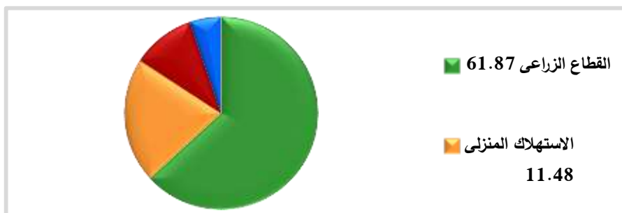
شكل (٣): استخدامات المياه في مصر بالمليار متر مكعب
