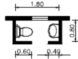
(شكل 17) مرحاض
