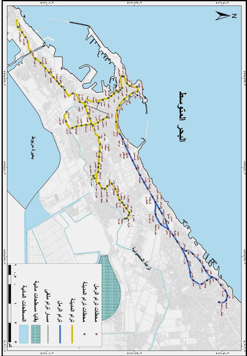
شكل (٤) : شبكة خطوط الترام بمحافظة الإسكندرية حتى عام ٢٠١٨.
