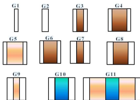
شکل (3): مقاطع الزجاج المستخدمة في مختلف الحالات
