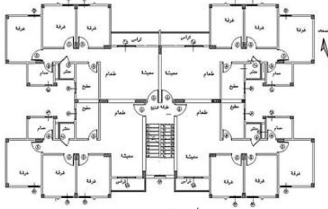
شكل (2): مسقط أفقي للمبنى المستخدم في الدراسة.
