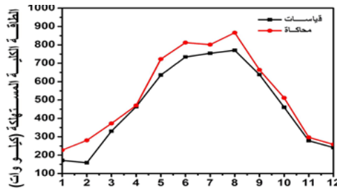
شكل (5): التحقق غير المباشر باستخدام نموذج الدراسة الذي حقق نسبة خطأ 10.28 %.
