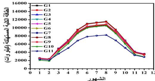
شكل (6): الاستهلاك السنوي للطاقة باستخدام أنواع الزجاج المختلفة في العزل.
