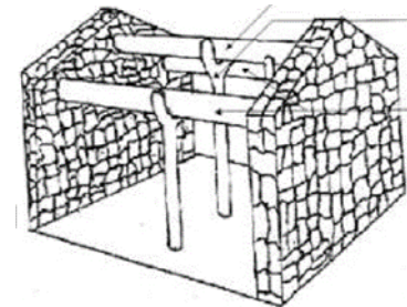
شكل (2) منظور يوضح الهيكل الانشائى للمسكن الاساسى (هجيرة 2016، 18)
