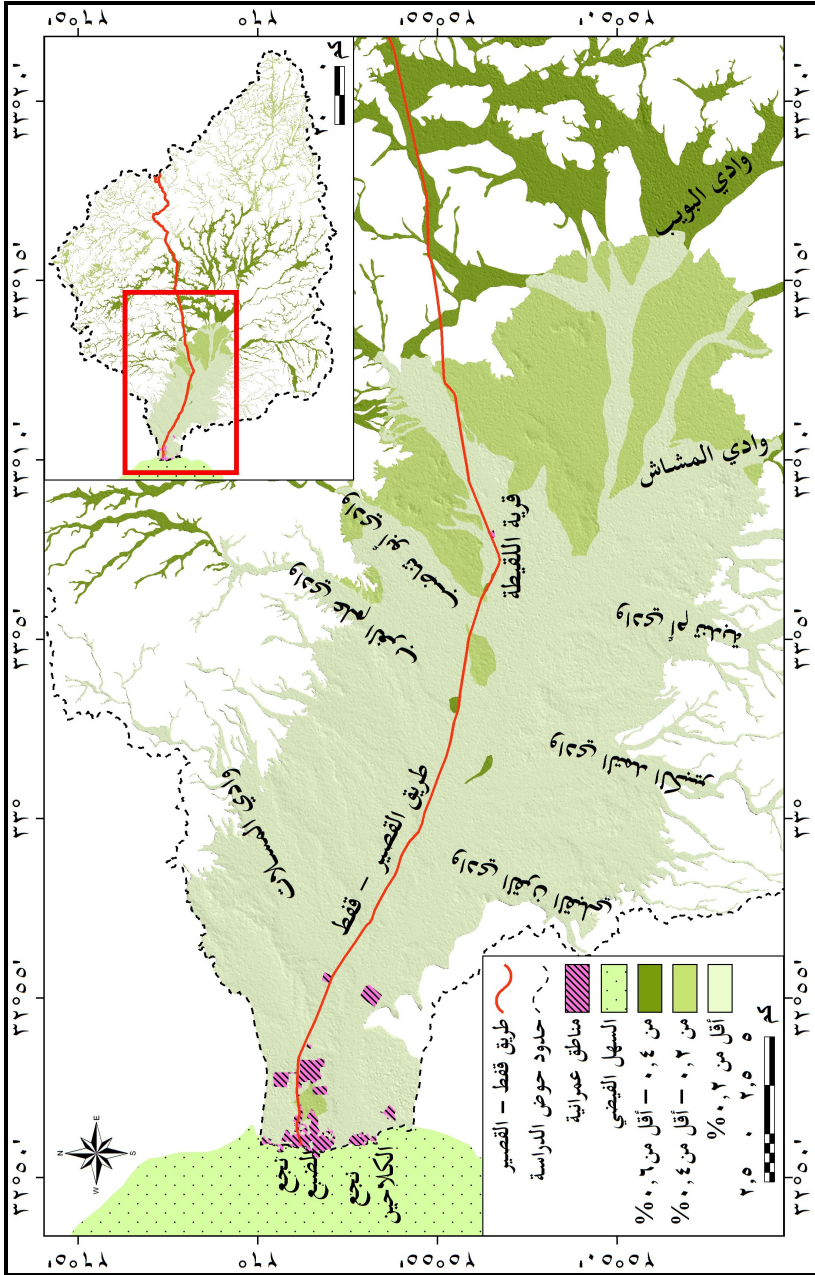
شكل (١٠) : التوزيع المكاني لنسبة المادة العضوية في تربة منطقة الدراسة.
