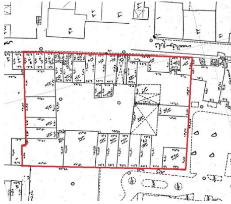
شكل (٣٠) مسقط أفقى لوكالة الزيت - عن مصلحة المساحة المصرية
