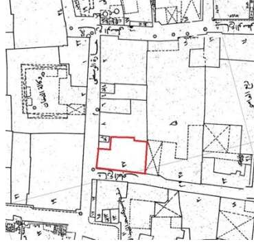
شكل (٤٠) مسقط أفقى لوكالة المغاربة - عن مصلحة المساحة المصرية
