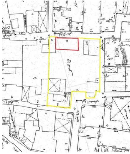
شكل (٣٨) مسقط أفقي لربع العاصي - عن مصلحة المساحة المصرية
