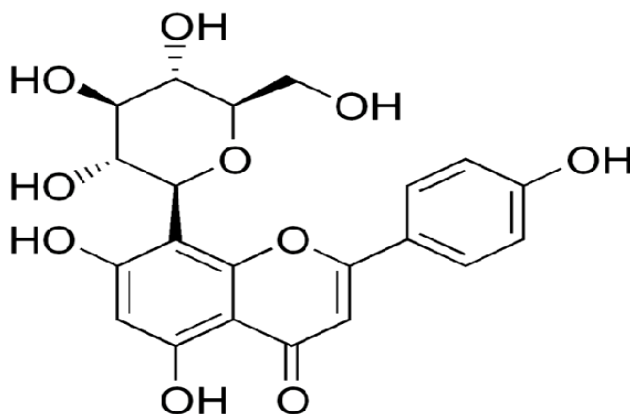
Vitexin (7)
