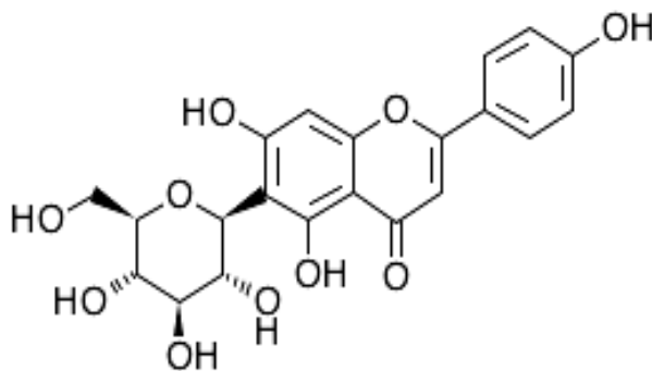
Isovitexin (6)
