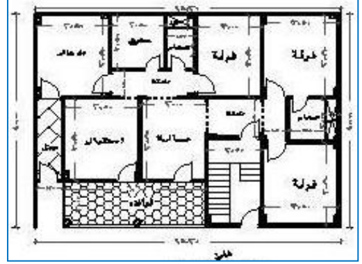
شكل (6) مساقط افقية لبعض المباني بالقرية المصرية بعد ثورة 25 يناير 2011
