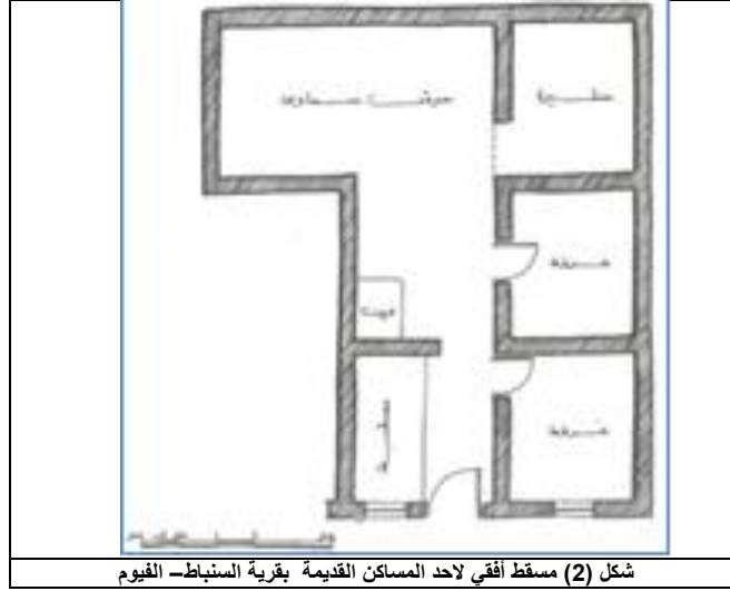
شكل (2) مسقط أفقي لأحد المساكن القديمة بقرية السنباط- الفيوم
