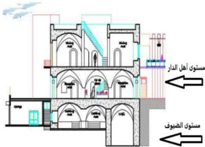
شكل "٧" قطاع رأسي في مبنى قصر الدويك ( المصدر: عمرو، سجاد، "إعادة تأهيل قصر دويك كمطعم تراثي فلسطيني"، كلية الهندسة المدنية والمعمارية، جامعة بوليتكنك فلسطين، ٢٠١٩م).
