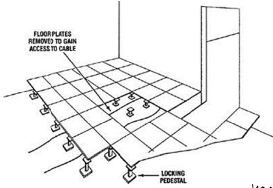
(شكل ٩) استناد لرفع الأرضية بالقدر المطلوب
