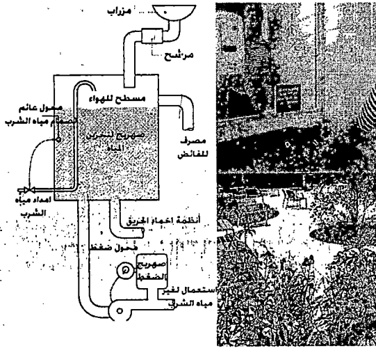
شكل ٣ بعض الأساليب المختلفة للحفاظ علي المياه، مستشفى لوثرن ادفوكات العام بولاية إلينوي، أمريكا. المصدر بتصريف: www.cannondesign.com
