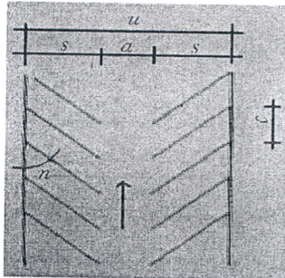
شكل (١٦): الأبعاد الأساسية لتصميم ساحة ركن السيارات. [13]
