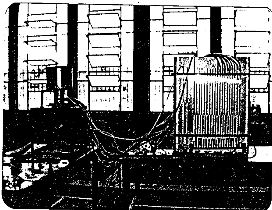
Fig.2. Test rig.
