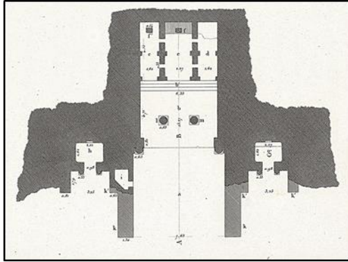
شكل 3: مخطط المعبد الكبير المقطوع في الصخر، سكييت. رسم: Cailliaud. Cailliaud 1821. Pl. V. Fig. 1.
