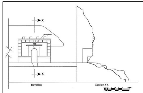
شكل 34: مخطط واجهة معبد بئر أبو سعفة. رسم: Mikhail. Sidebotham. S.E.. et al. 2004b. p.
