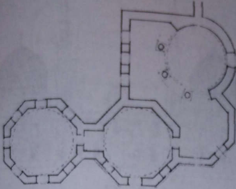
شكل رقم (٤٩) قبتى تربة سمبل أفندي بالأناضول
