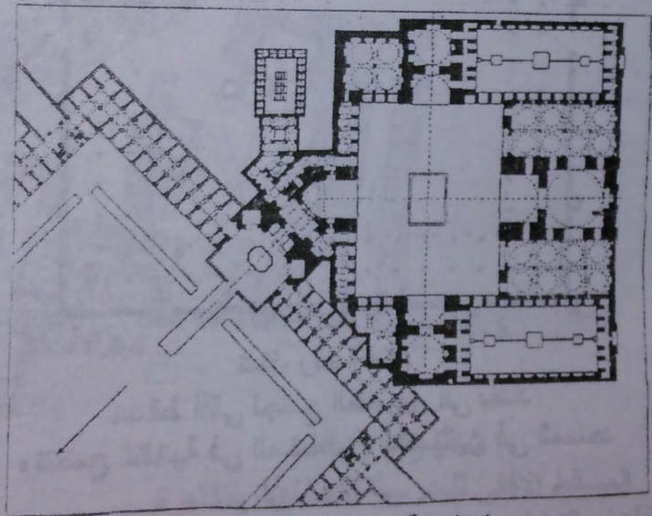
شكل رقم (١٩) مسقط أفقي لمسجد الشاة بمدينة أصفهان عن بوب
