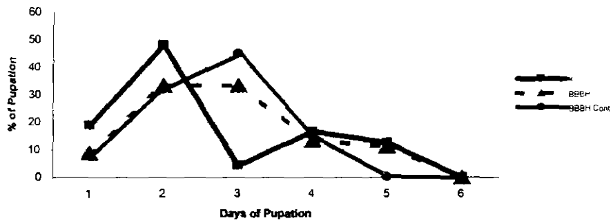
Fig. 4. a. BBBH
