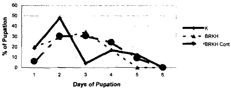
Fig. 4.c. BRKH
