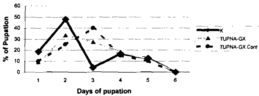
Fig. 4.b. Tinopal UPNA-GX
