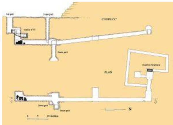
مسقط المساكن الجنائزية لسنوسرت الثاني
