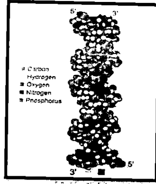
شكل رقم (٦) يوضح التركيب الدقيق لجزئ الـ DNA (٥٧)
