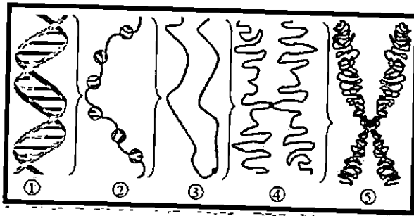
شكل رقم (١) أشكال مختلفة لحمض النووي (DNA) وكذلك الكروموسومات (١٨)
