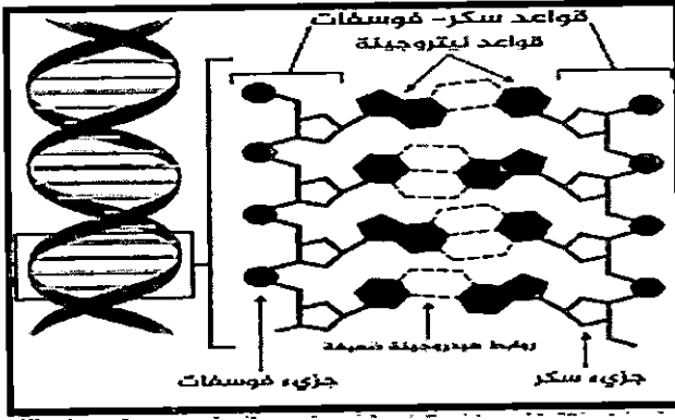
شكل رقم (٤) يوضح مكونات الدنا D.N.A (الجين) (٥٥)
