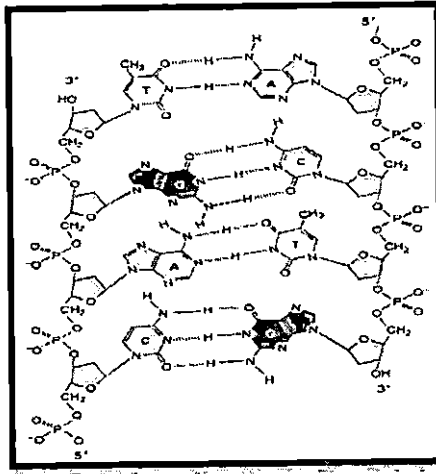
شكل رقم (٥) يوضح التركيب التفصيلي لسلاسل البيولي نيوكليوتيد (٥٦)
