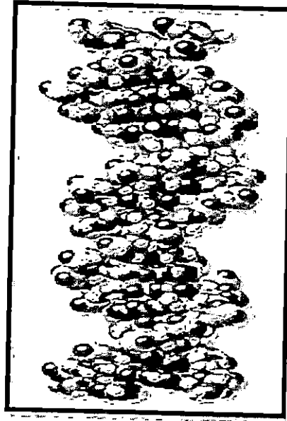
شكل رقم (١٩) يوضح الفراغ الخارجي لجزئ DNA (٨٣)
