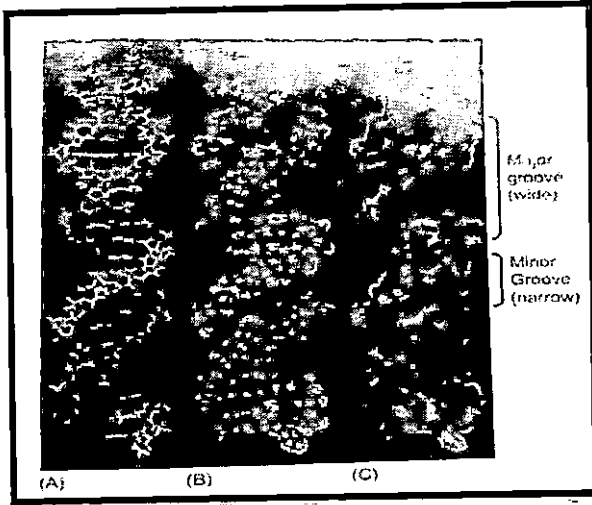
شكل رقم (٢٠) يوضح الفراغ الداخلي والخارجي في الدنا (٨٤)
