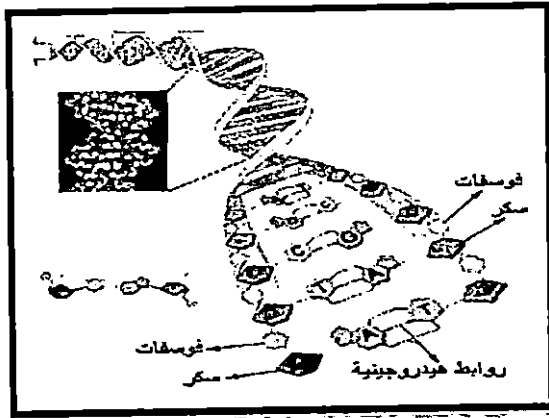
شكل رقم (٢) يوضح التركيب الدقيق لجزئ الدنا DNA الحلزوني (٥١)
