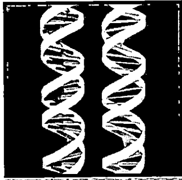
شريط الـ DNA
