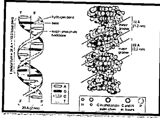
شكل رقم (٢) يوضح الشكل الحلزوني لجزئ الدنا DNA (٥٢)
