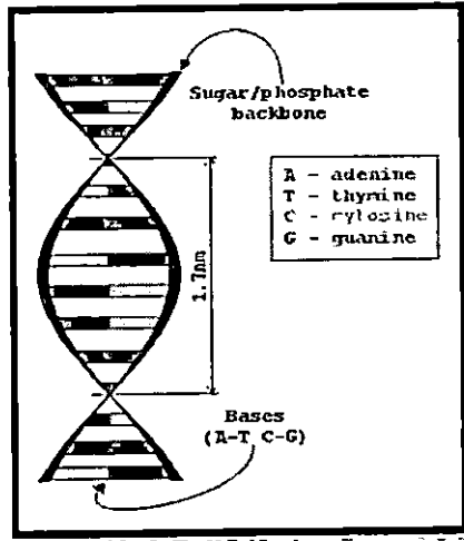
شكل رقم (١٧) يوضح الفراغ الداخلي المغلق داخل جزئ الـ DNA (٨١)
