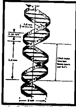
شكل رقم (٢٢) يوضح التناسب في شريط الـ DNA
