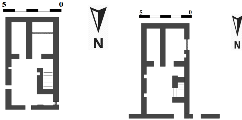
شكل (٤) المسقط الافقي للطابق الارضي لمنزل أحمد سفر بالهنداو - عمل الباحثة
