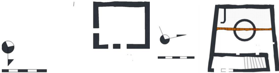
شكل (٦) المسقط الافقي لطاحونة حارة الجامع بالهنداو - عمل الباحثة
