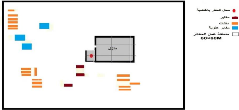
كروكي يوضح منطقة الحفائر بالشغب وماتم العثور عليه موسم ٢٠١٦
