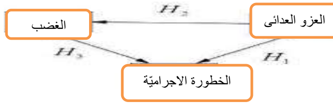
شكل (١-١). مقترح معاملات المسارات للمتغيرات الدراسة.
