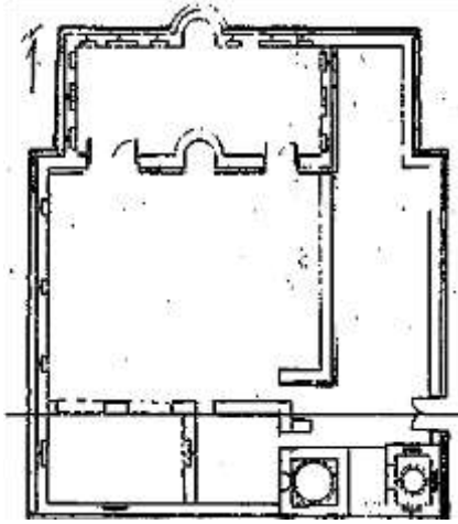
(شكل ١٣) يوضح تخطيط المدرسة المنصورية العليا بمدينة زبيد عن مكايي، هيفاء عبد القادر، "مدارس اميرات الدولة الرسولية ٦٢٦ - ٨٥٨ هـ / ١٢٢٨ - ١٤٥٤ م، دراسة اثرية معمارية"، أطروحة دكتوراه، كلية الاداب/ جامعة عدن، ٢٠١٣ م، ٣٤٤.
