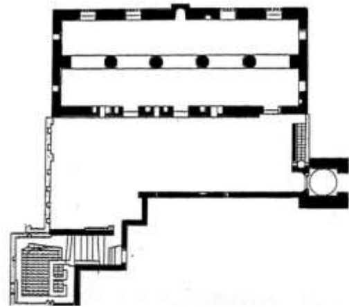
(شكل ١٨) يوضح تخطيط المدرسة المزجاجة بمدينة زبيد، عن: عثمان، "المدرسة"، ١٧٧.
