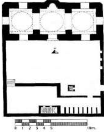
(شكل ٥) يوضح تخطيط مدرسة جمال الدين الريمي بمدينة زبيد، عن: عثمان، محمد عبده، "المدرسة في زبيد ٦٢٦_٨٥٨/١٢٢٨م ١٤٥٤م تخطيطها وعمارتها"، رسالة ماجستير، كلية الاداب/ جامعة بغداد، ١٩٩٢م، ١٧٤.
