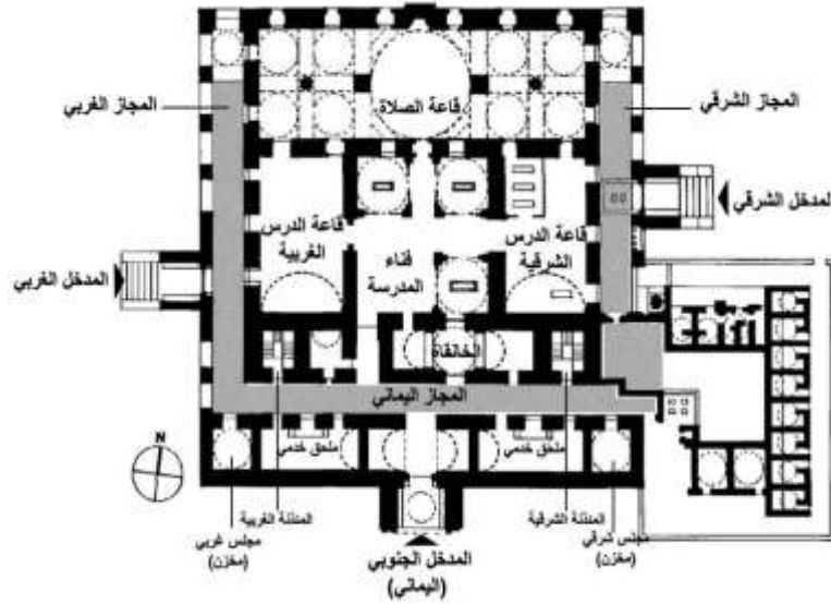
(شكل ١) يوضح تخطيط المدرسة الأشرفية نقلا عن:
