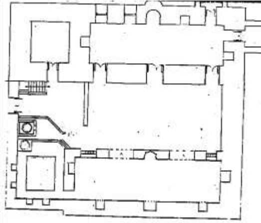
(شكل ١٧) يوضح تخطيط المدرسة المحالية بمدينة زبيد، عن: عثمان، "المدرسة"، ١٧٦.
