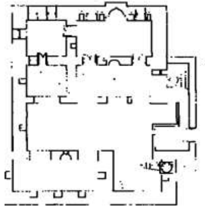
(شكل ١٩) يوضح تخطيط المدرسة الياقوتية بمدينة زبيد عن: SADEK, «Patronage», 520.
