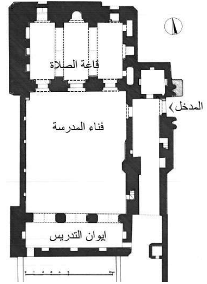
(شكل ١٢) يوضح تخطيط المدرسة الفرحانية بمدينة زبيد، عن: عثمان، "المدرسة"، ١٧٨.
