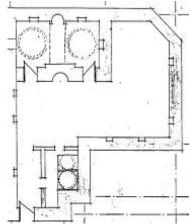
(شكل ١٠) يوضح تخطيط المدرسة الدعاسية بمدينة زيد، عن: عثمان، "المدرسة"، ١٧٠.
