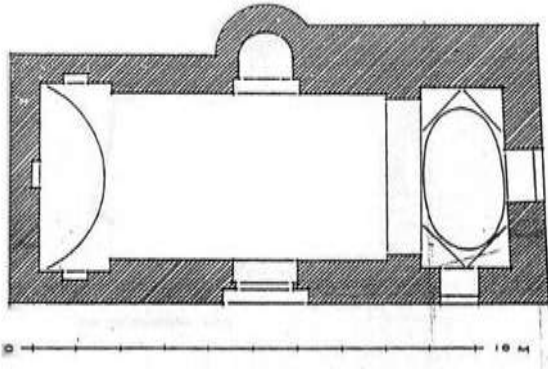
(شكل ١١) يوضح تخطيط المدرسة الفاتنية بمدينة زيد، عن: عثمان، "المدرسة"، ١٧٣.
