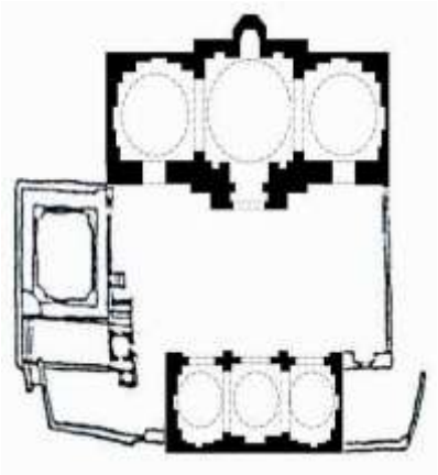
(شكل ٧) يوضح تخطيط المدرسة الياقوتية بحيس عن: الحداد، عبد الله عبد السلام، مدينة حيس تاريخها واثارها الدينية، القاهرة: دار الأفاق العربية، ١٩٩٩م، ٤١٢، شكل ٥٩.
