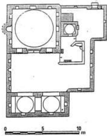
(شكل ٩) يوضح تخطيط المدرسة التاجية بمدينة زيد بمدينة زيد، عن: عثمان، "المدرسة"، ١٦٩.
