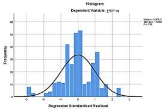
شكل (٢) : التوزيع الطبيعي للبيانات
