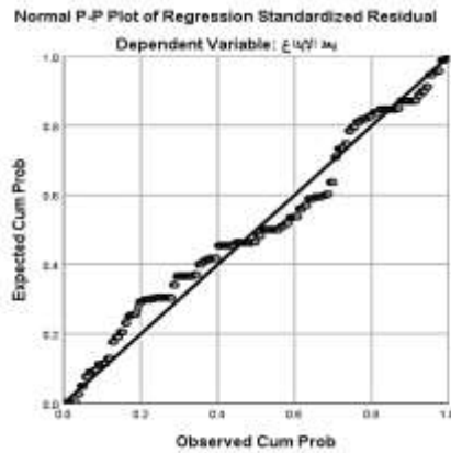
شكل (٣) : Normal P-P plot
