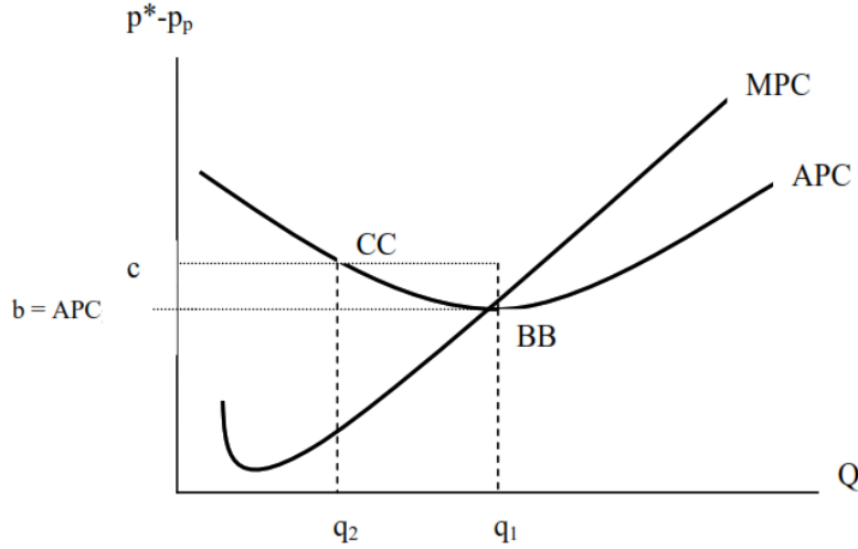
شكل (2) التكلفة والنتاج الحدي لعملية حلج القطن
