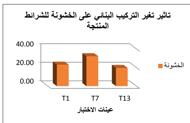
شكل (14) نتائج اختلاف التركيب البنائي على خاصية الخشونة للشرائط المنتجة باستخدام 1/150 دينير بوليستر محلول للسداء واللحمة
