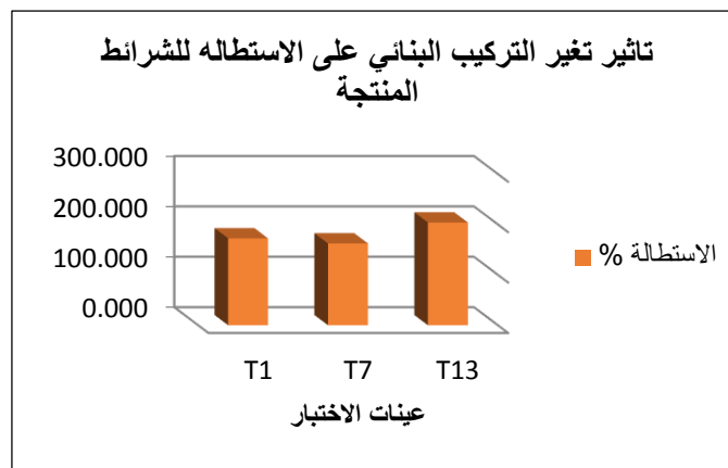
شكل (12) نتائج اختلاف التركيب البنائي على خاصية الاستطالة (%) للشرائط المنتجة باستخدام 1/150 دينير بوليستر محلول للسداء واللحمة
