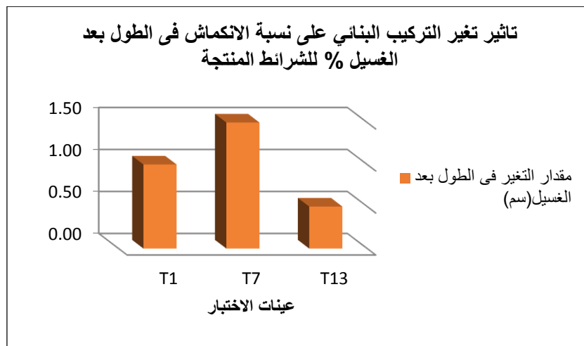
شكل (16) نتائج اختبار اختلاف التركيب البنائي على نسبة الانكماش في الطول بعد الغسيل % للشرائط المنتجة باستخدام 1/150 دينير بولستر محلول للسداء واللحمة
