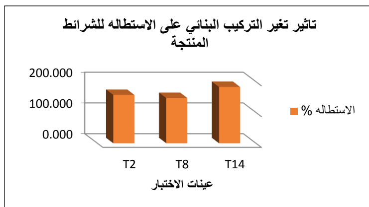
شكل (13) نتائج اختلاف التركيب البنائي على خاصية الاستطالة (%) للشرائط المنتجة باستخدام 1/150 بوليستر للسداء و 1/30 قطن للحمة
