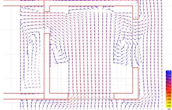
شكل (١٣) محاكاة لحركة الهواء داخل الغرفة الأولى موضحة باسهم توضح اتجاه حركة الهواء ومسارها وتوزيعها داخل الغرفة
