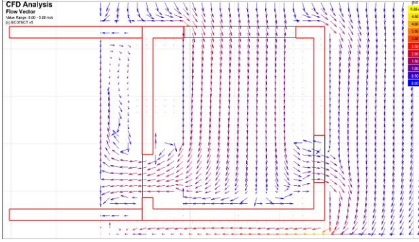
شكل (١١) محاكاة لحركة الهواء داخل الغرفة الأولى موضحة بأسهم توضح اتجاه حركة الهواء ومسارها وتوزيعها داخل الغرفة
