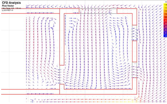
شكل (١٥) محاكاة لحركة الهواء داخل الغرفة الأولى موضحة باسهم توضح اتجاه حركة الهواء ومسارها وتوزيعها داخل الغرفة
