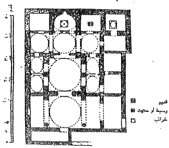
كنيسة نقادة د كما رسمها سير آرثر جوردن
