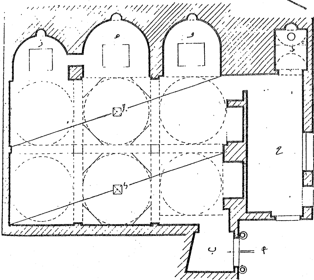
شكل (٤) رسم تخطيطي لكنيسة الأمير تادرس المشرقي.
