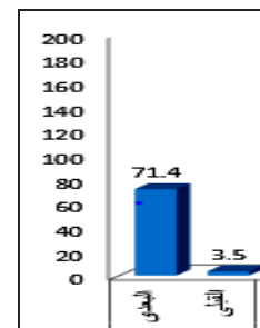
شكل (2) : نتائج اختبار (ت) للعينات المترابطة للفروق بين متوسطات درجات اختبار الأداء المهاري (القبلي – البعدي) يتضح من الجدول و الشكل السابقين أن :
