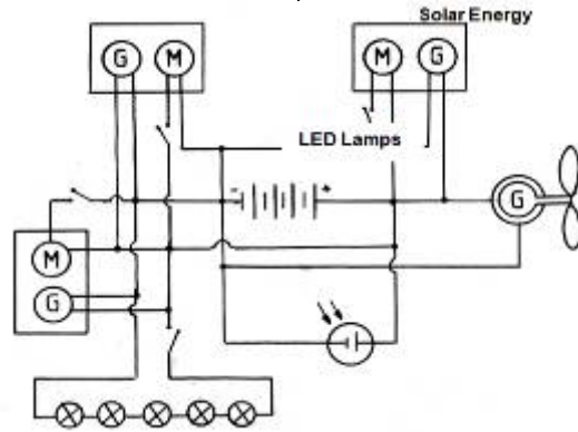
شكل ( 4 ) يوضح وحدة توصيل الطاقة ذات الاربعة اطراف
