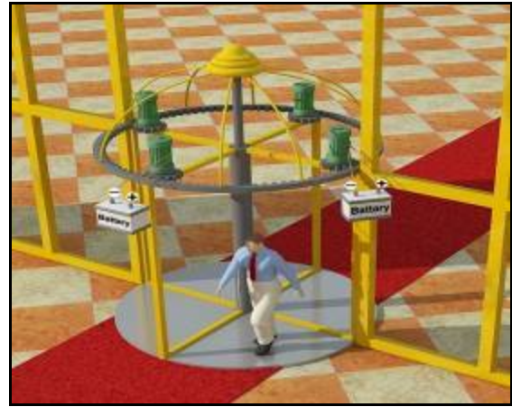
شكل ( 10 ) يوضح كيفية الاستفادة من الباب الدوار في توليد الطاقة
