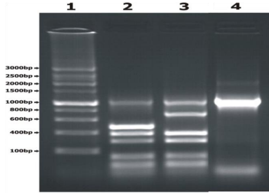
الشكل 1: تمييز السلالات البكتيرية المستخدمة باستخدام تفاعل البلمرة متعدد الشدف ( Multiplex PCR ).
