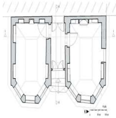
شكل (٩) مؤقتخانه ومكتبة كويرلو محمد باشا- بسفرنبلو- - نقلاً عن:
